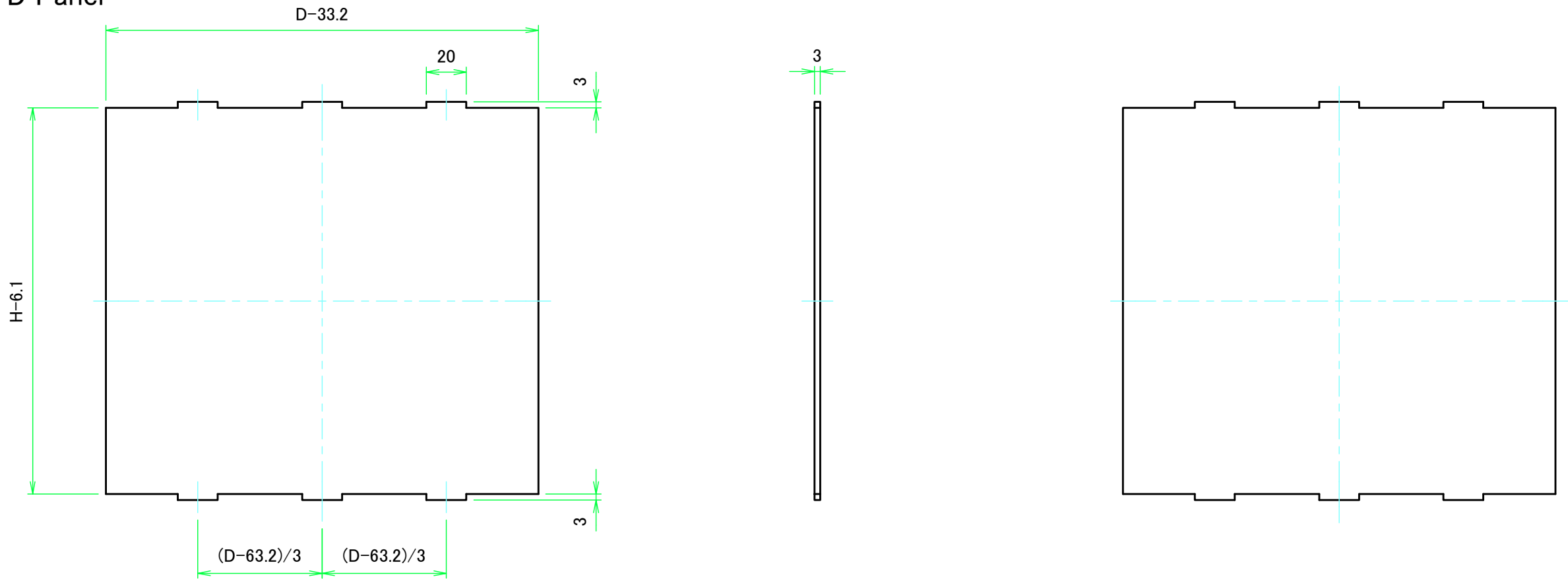
Dパネル1表面 / D Panel 1 Frontside
