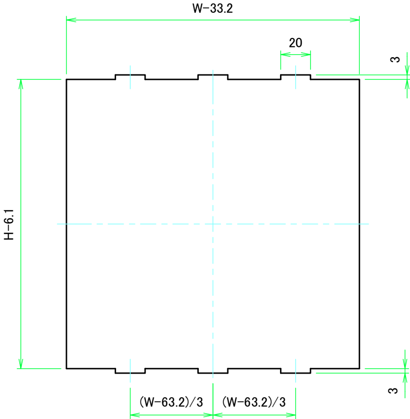
Wパネル1表面 / W Panel 1 Frontside
