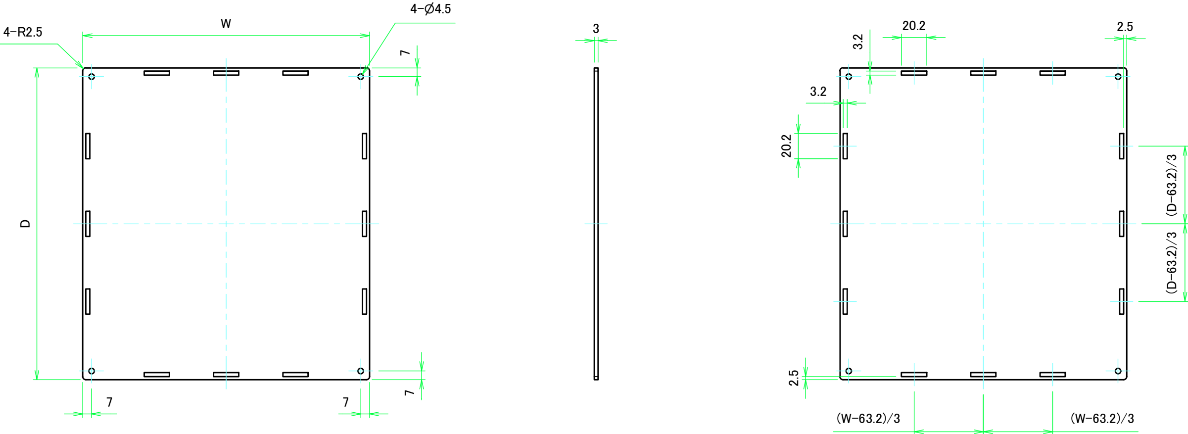
上カバー表面 / Top cover Frontside
